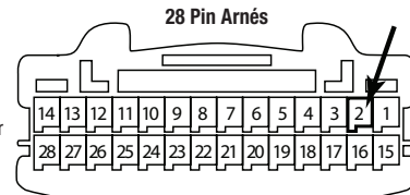
Esta es la vista de cable del conector en el vehículo
